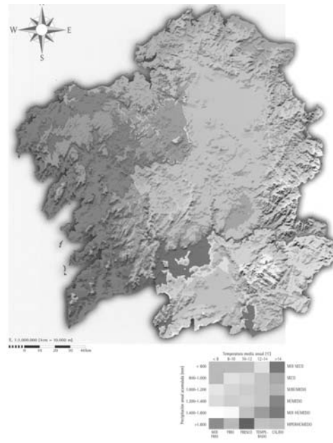
Figura 10.- Regímenes ombrotérmicos de Galicia según Martínez Cortizas & Pérez Alberti (1999)
